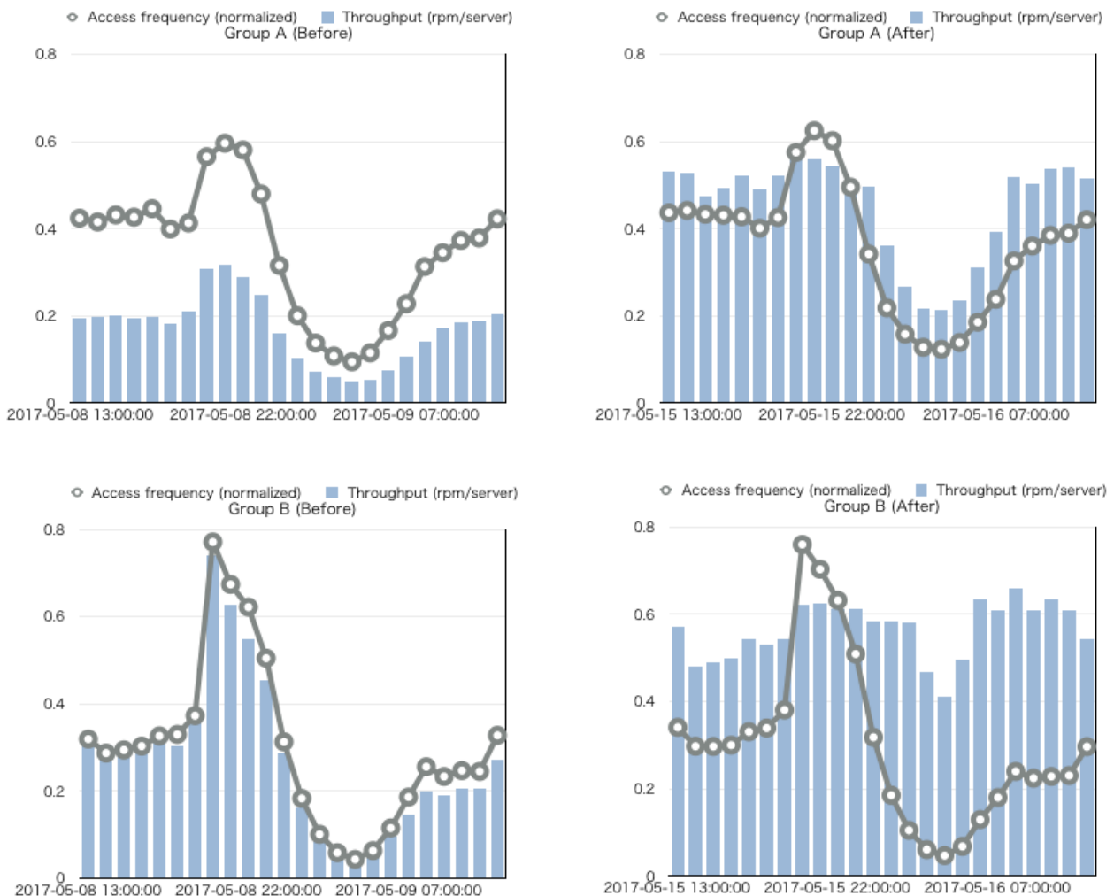
図5 アクセス頻度の推移
