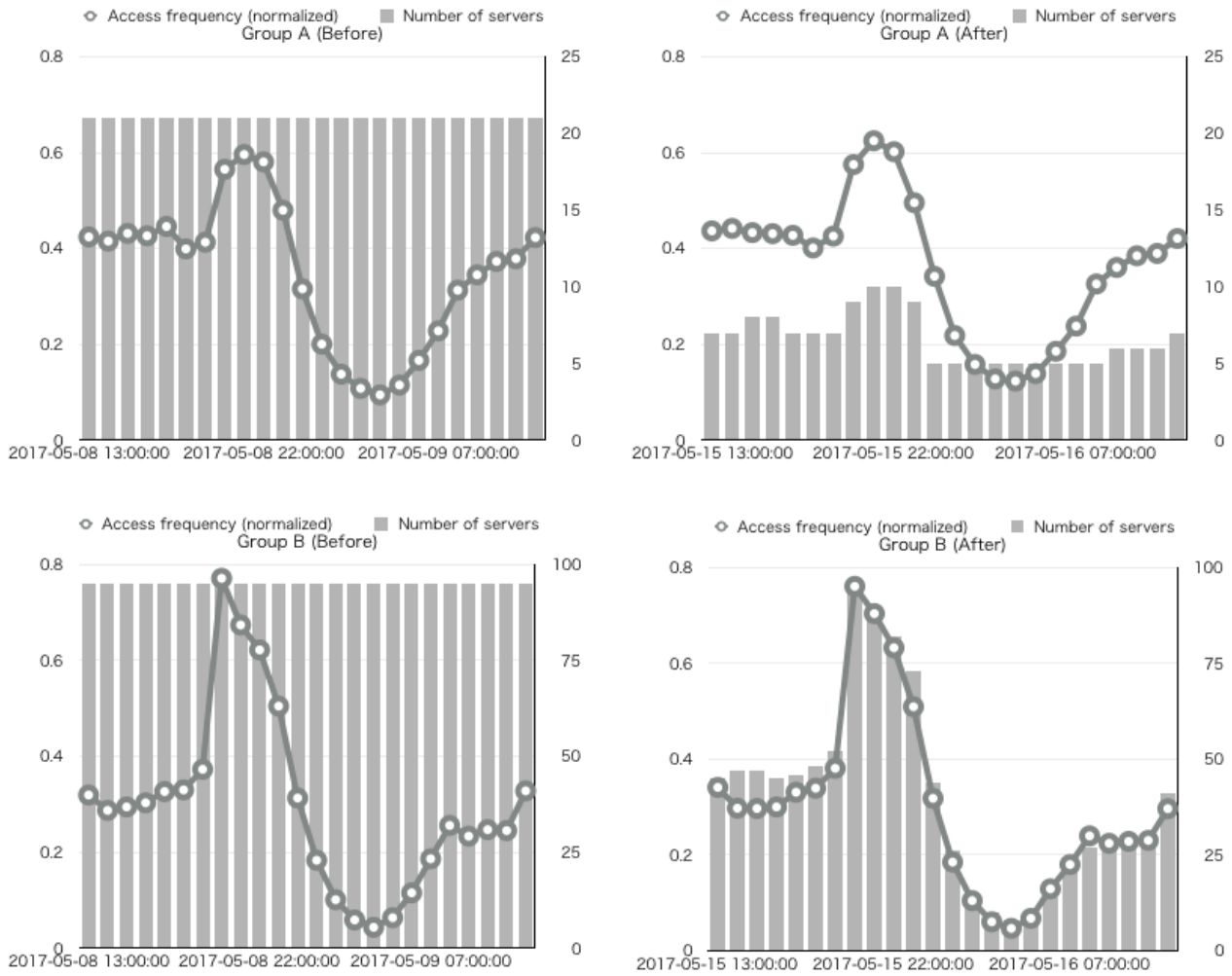
図4 仮想サーバ台数の推移
