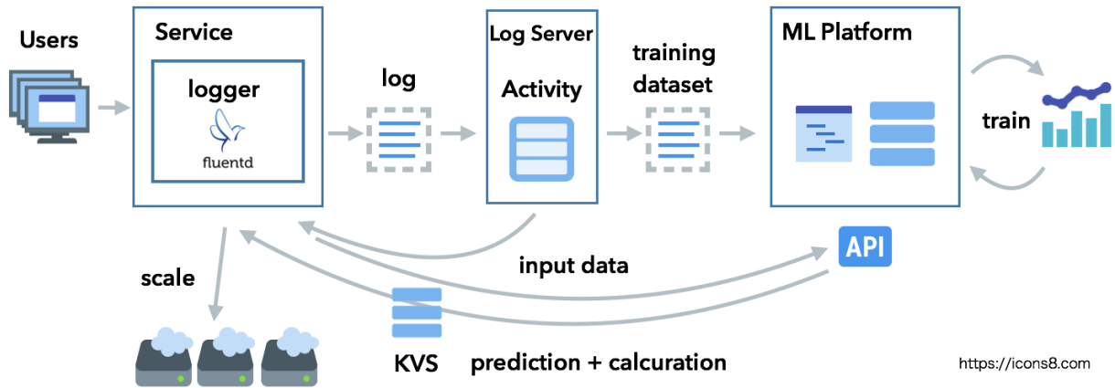
図2 アクセス頻度予測と仮想サーバ台数算出の処理フロー
