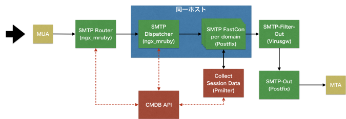
図 6 SMTP 送信フロー Fig. 6 SMTP Send Flow
