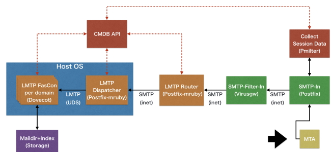
図 4 SMTP 受信フロー
