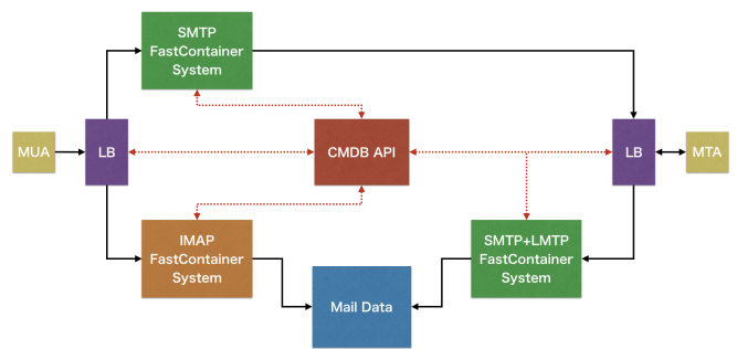
図 3 提案するメールシステムの全体フロー
